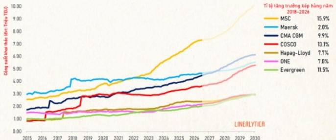
Công suất vận tải 2015-2026 và dự báo đến 2030 của Top 7 hãng tàu toàn cầu
